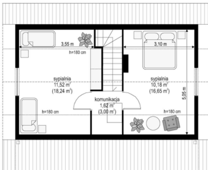
Rzut poddasza
