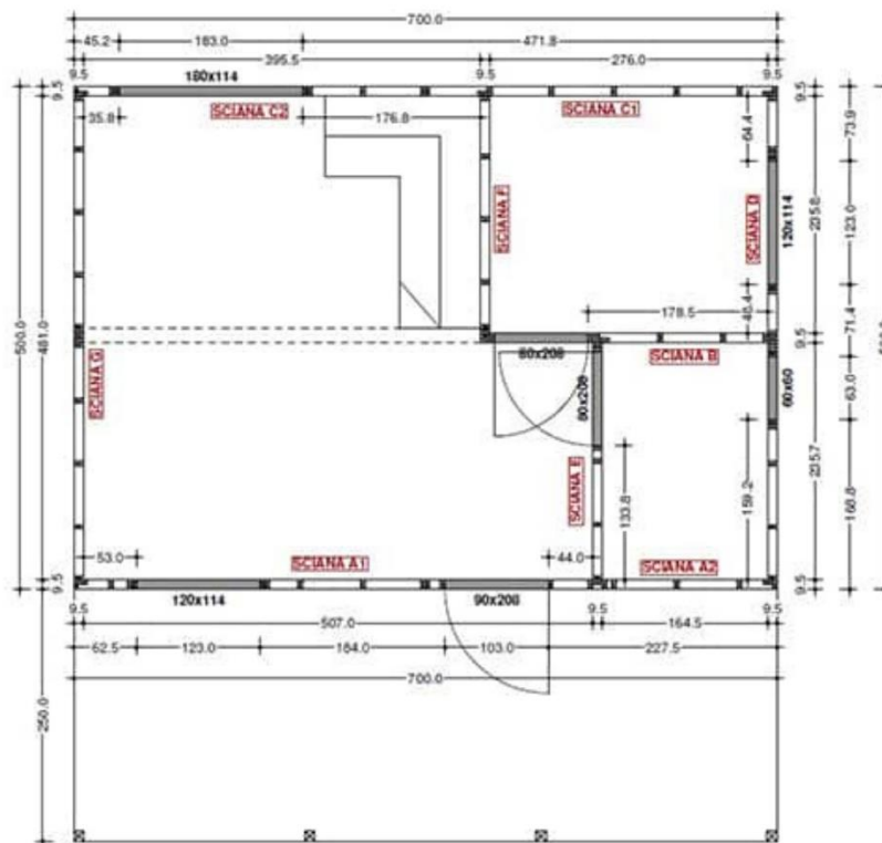
Rzut poddasza
