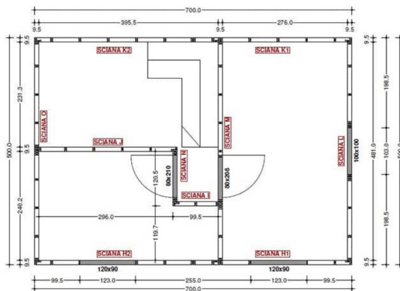
Rzut poddasza
